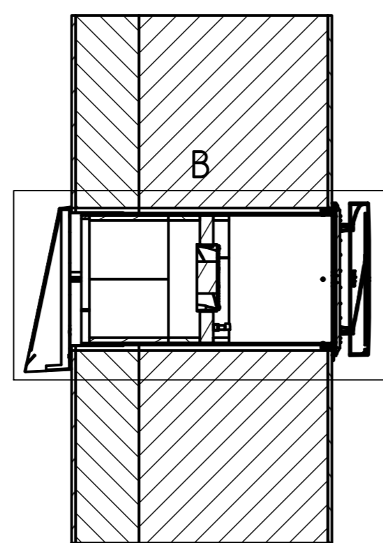
A-A ( 1 : 10 )
