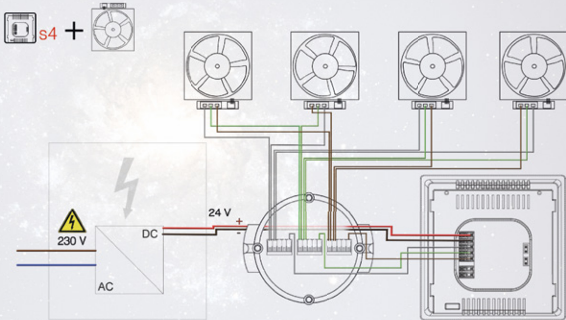
Anschlussbeispiel sternförmiger Anschluss
