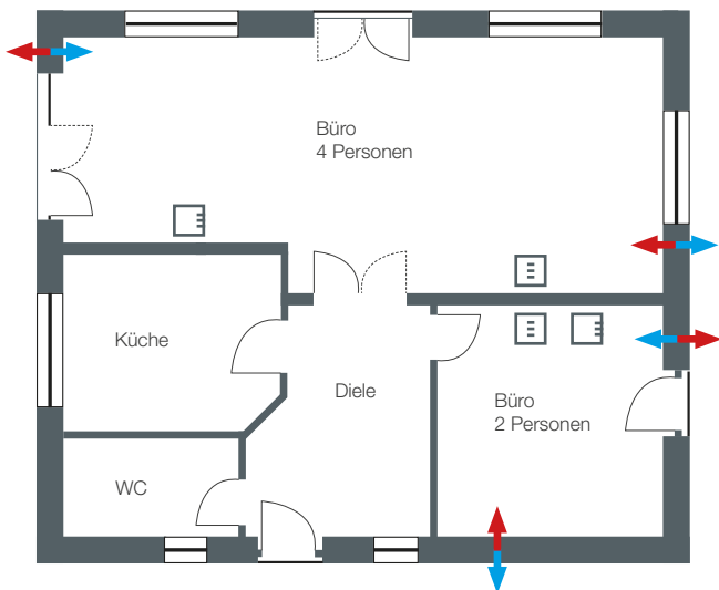
Beispiel Bürolüftung mit 2 Office-Sets:
